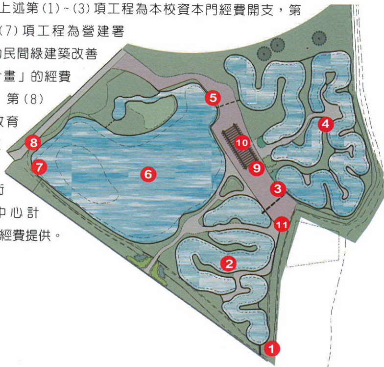
圖3 本校人工濕地系統的平面圖，1：污水進流口，2：表面下流動（SSF）濕地，3：SSF濕地出口，4：表面流動（FWS）濕地，5：FWS濕地出口，6：景觀生態池，7：生態池出口，8：水回收再利用高壓幫浦及管線，9：太陽能光電設施，10：休憩花架，11：氣象及水文監測站，淺紫色區域則為透水鋪面鋪設範圍。
